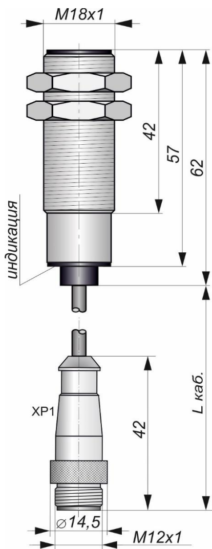
Габаритный чертеж
